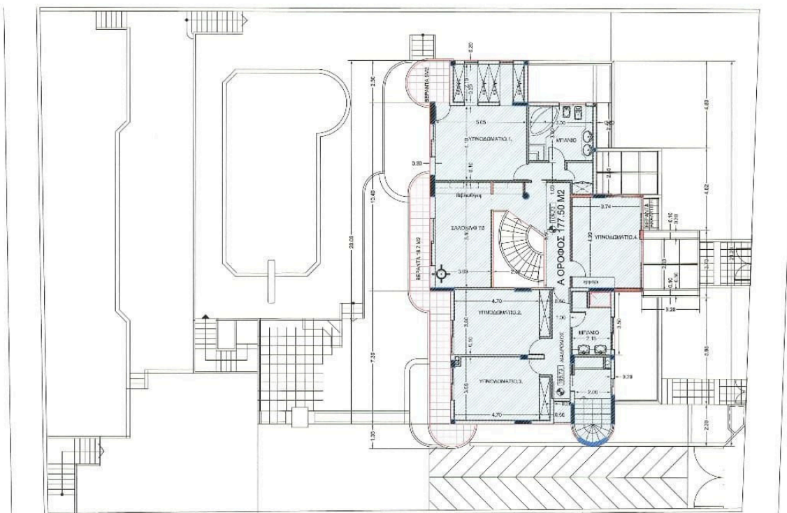
ΚΑΤΟΨΗ ΟΡΟΦΟΥ
