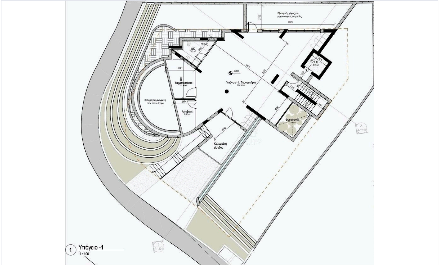
A Ισόγειο 1:100
