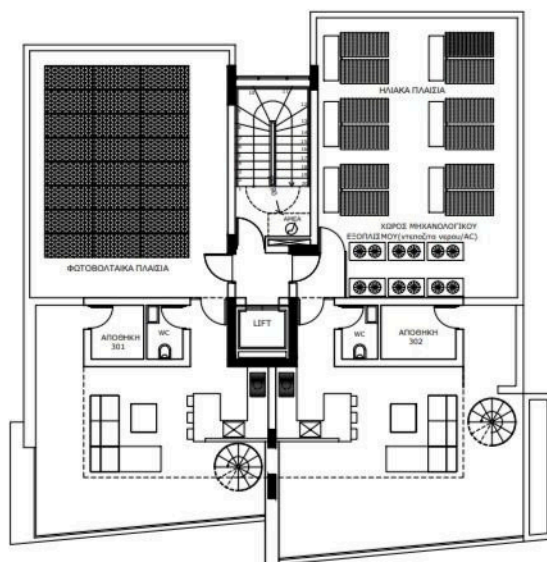
ΚΑΤΟΨΗ ΟΡΟΦΗΣ
