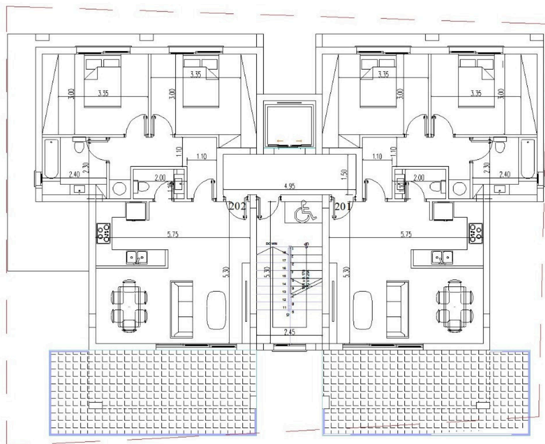
ΚΑΤΟΨΗ 2ου ΟΡΟΦΟΥ
