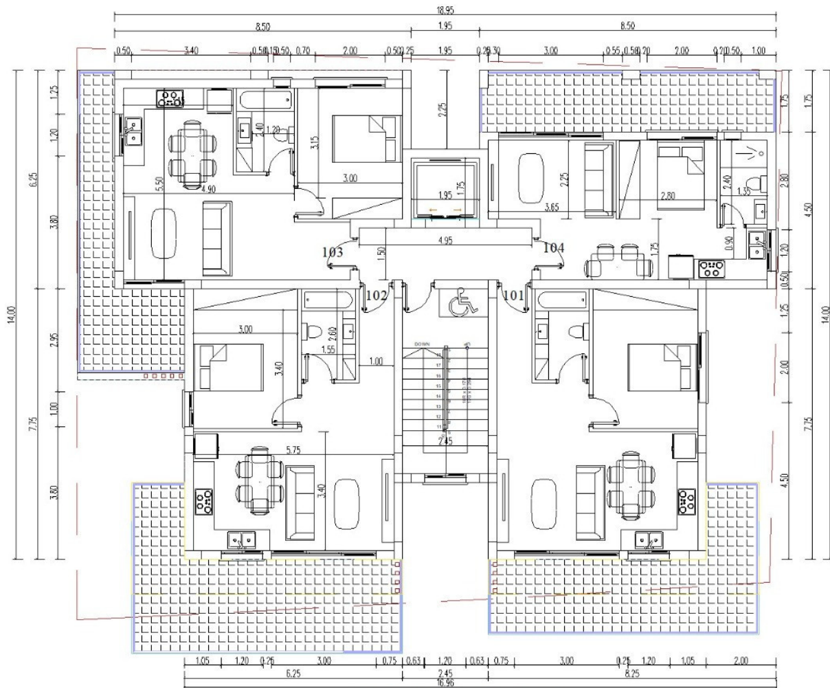
ΚΑΤΟΨΗ 1ου ΟΡΟΦΟΥ
