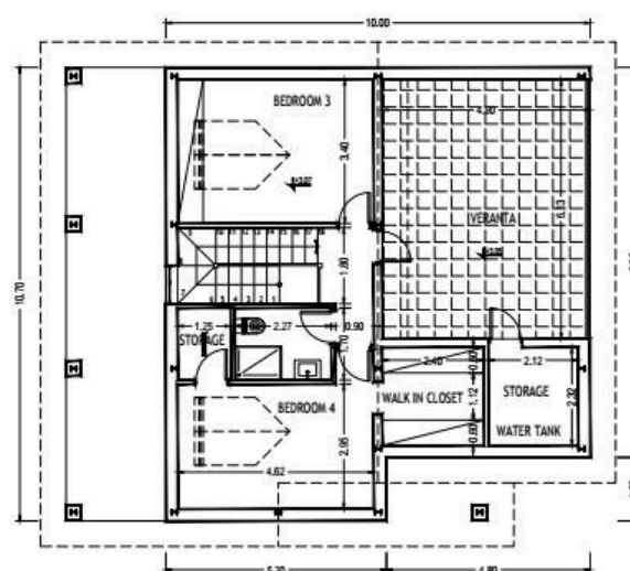
ΚΑΤΟΨΗ ΣΟΦΙΤΑΣ ΚΛΙΜΑΚΑ 1:100
