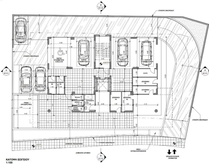
KATΩH ΙΣΤΕΓΙΩY 1:100
