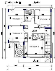
ΚΑΤΩΦΗ ΟΡΟΦΟΥ
