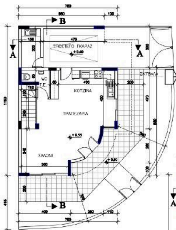
ΚΑΤΟΨΗ ΙΣΟΓΕΙΟΥ
