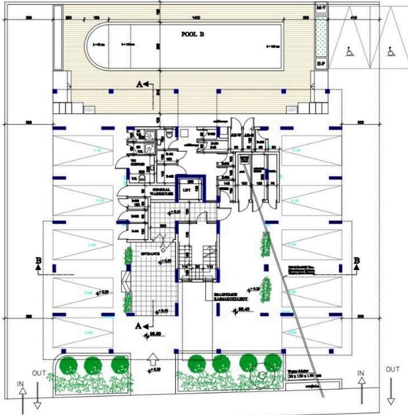
ΚΑΤΩΦΗ ΙΣΟΓΕΙΟΥ BLOCK B
