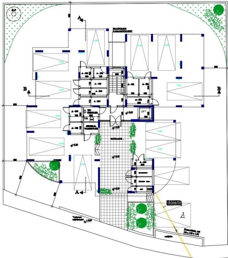
ΚΑΤΟΨΗ ΙΣΟΓΕΙΟΥ BLOCK A
