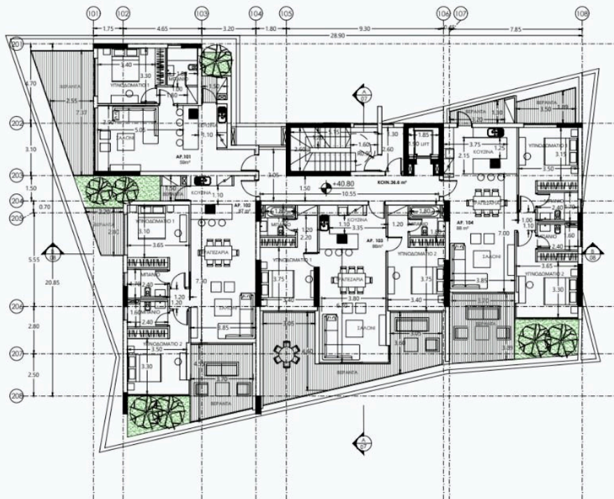
ΚΑΤΟΨΗ 3ΟΥ ΟΡΟΦΟΥ
