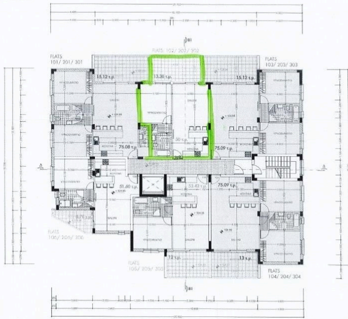
ΚΑΤΟΨΗ 1ου,2ου,3ου
